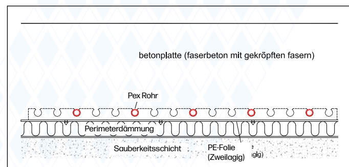
Beispiel: Rohrbefestigung auf der Perimeterdämmung
